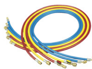
Juego de 3 mangueras GOODYEAR 900 mm 5/16\" HSAE x 5/16\" HSAE con llaves de bola
